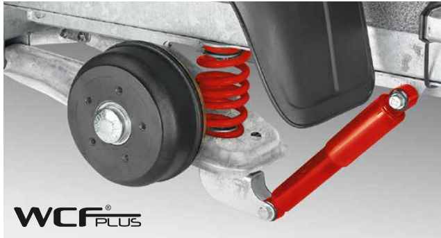
Rijcomfort dankzij het World-Class-chassis volgens automobielstandaard met wiel-schokbreker en Tempo 100-ontheffing (geldt uitsluitend voor Duitsland).
