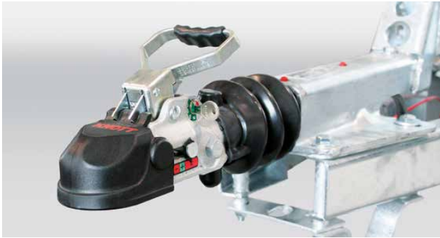
Sicheres An- und Abkuppeln durch die abschließbare Gusskupplung mit gummiertem, komfortablem Herzgriff und Soft-Top (Anfahrerschutz).
